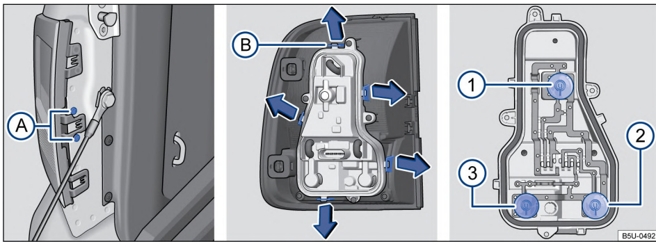
Fig. 172 Luz trasera: C desmontar el portalámparas y ①, ②, ③, ④ y ⑤ desmontar las bombillas.
