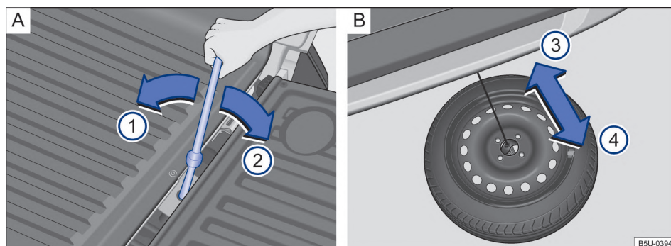
Fig. 199 A En el compartimento de carga: acceso a la rueda de emergencia. B Debajo del vehículo: rueda de emergencia totalmente en el piso y extracción de debajo del vehículo.
