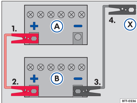
Fig. 184 Esquema para la conexión de los cables de arranque auxiliares de arranque: batería del vehículo descargada (A) y batería del vehículo que provee la corriente (B).
