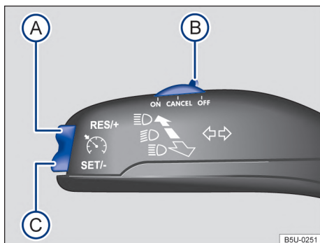
Fig. 86 A la izquierda, en la columna de dirección: palanca con interruptor y teclas de mando del GRA.
