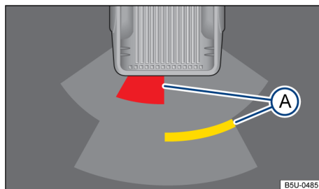
Fig. 89 Presentación del display del control de distancia de estacionamiento (display a color): A obstáculo reconocido en el segmento.
