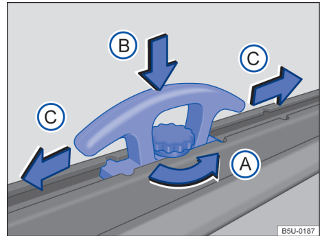
Fig. 154 En el compartimento de carga: soporte deslizante para vehículos sin capota marítima.
