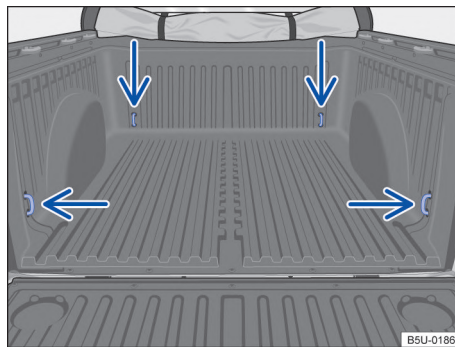
Fig. 152 Compartimento de carga: ojales de amarre.
