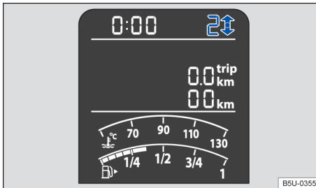
Fig. 78 En el panel de instrumentos: indicador de cambio de marcha (variante 1).
