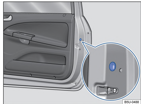
Fig. 44 En la parte delantera de la puerta derecha: bloqueo de emergencia, cubierto por una junta de goma.
