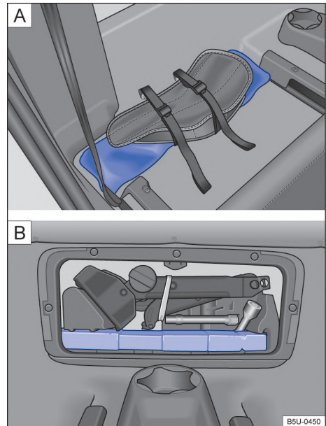
Fig. 38 [A] Atrás del asiento del pasajero: triángulo de seguridad. [B] En el piso del asiento trasero: triángulo de seguridad - Nueva Saveiro Doble Cabina.
