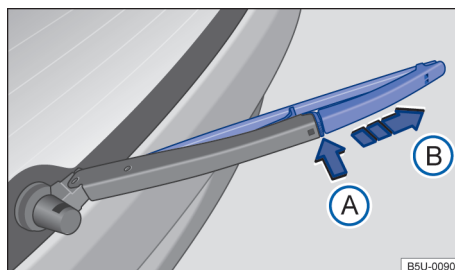
Fig. 168 Sustituir la escobilla limpiaparabrisas de la luneta trasera.
