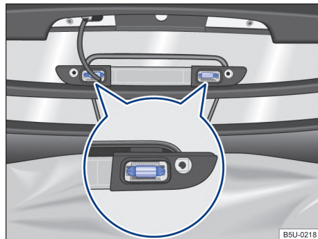
Fig. 176 Linterna de freno elevada: remover la lámpara incandescente de iluminación del compartimento de carga.
