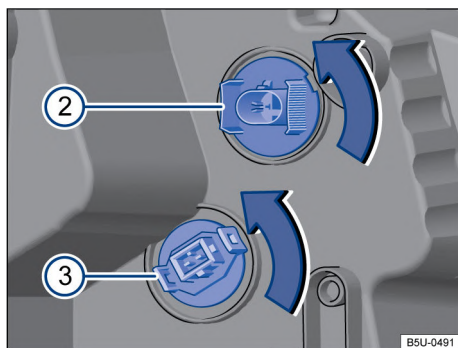
Fig. 170 En el vano motor: vista trasera del faro delantero 2 luces diurnas / luz de posición y 3 indicadores de dirección.
