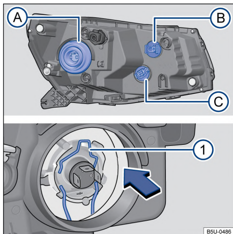
Fig. 169 En el vano motor: vista trasera del faro delantero con cubierta de goma (lado izquierdo de la ilustración) - A luz de cruce / luz de carretera B luz de conducción / luz de posición y C indicadores de dirección. Vista trasera del farol delantero sin cubierta de goma (lado derecho de la ilustración): 1 resorte de bloqueo de la lámpara incandescente del farol bajo/farol alto.
